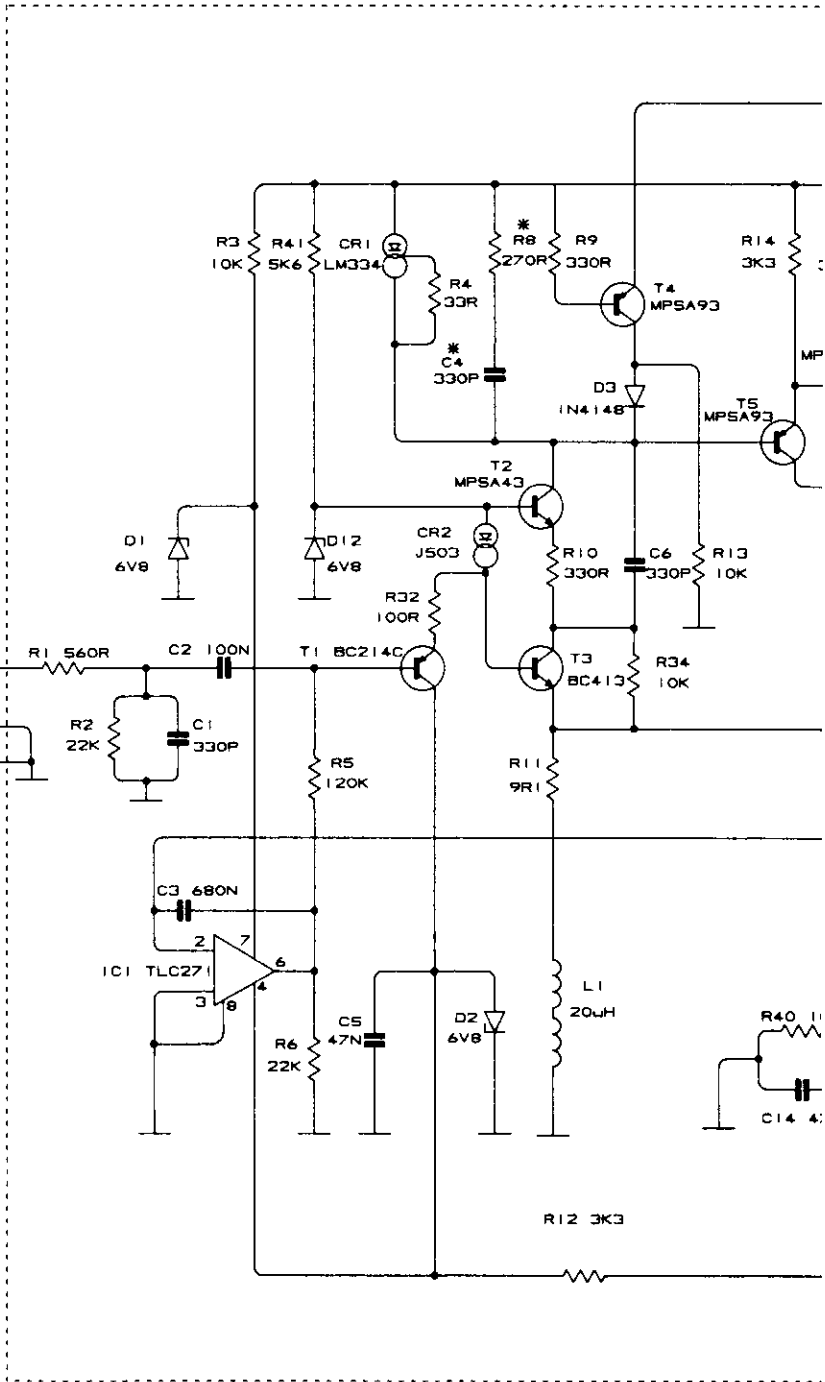
OPTIONAL ACTIVE FLOATING INPUT MODULE
