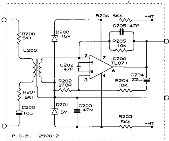
OPTIONAL ACTIVE FLOATING INPUT MODULE
